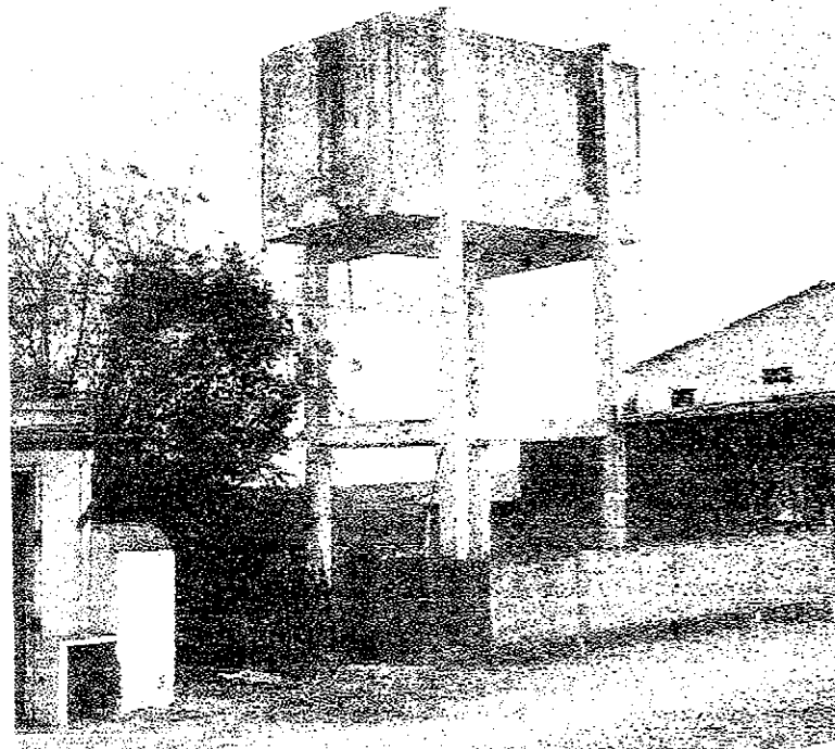
Níveis de sustentação do reservatório elevado em processo de corrosão avançada.
