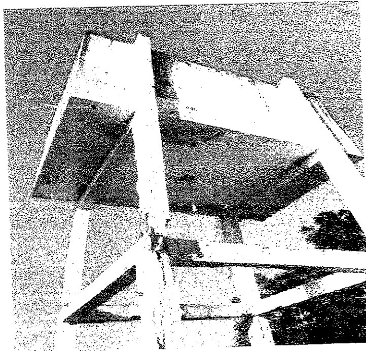
- Pilares de sustentação do reservatório elevado em processo de corrosão avançada.
