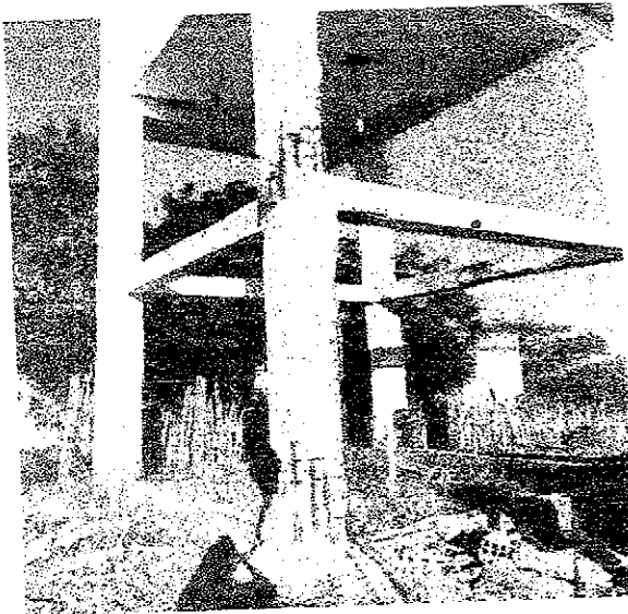
- Pilares de sustentação do reservatório elevado em processo de corrosão avançada.
