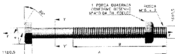
VISTA LATERAL
