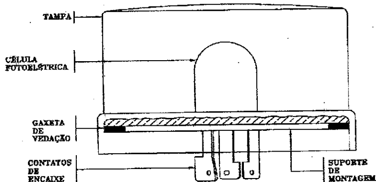
VISTA LATERAL
