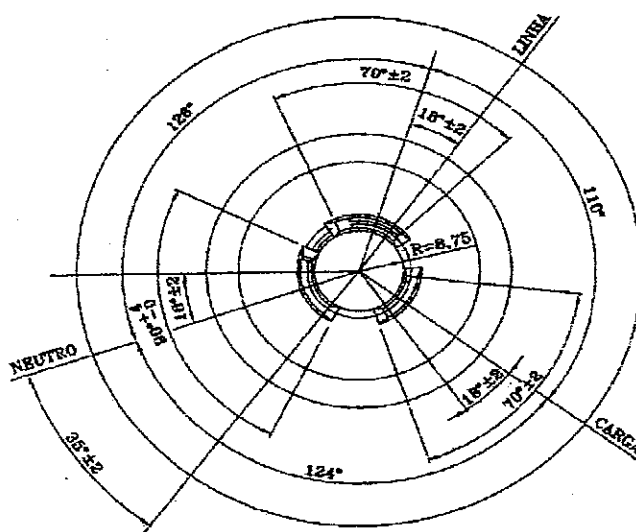
VISTA INFERIOR
